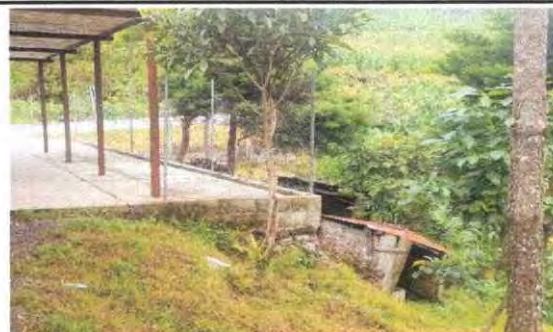
Foto 12: Colocación y Reforzamiento de muro de contención 20mts. Lineal.
